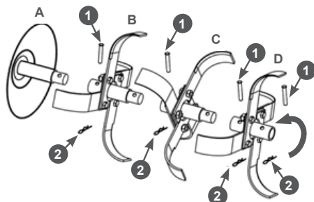
Рис. 3 Установка фрез
